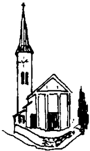
Au
